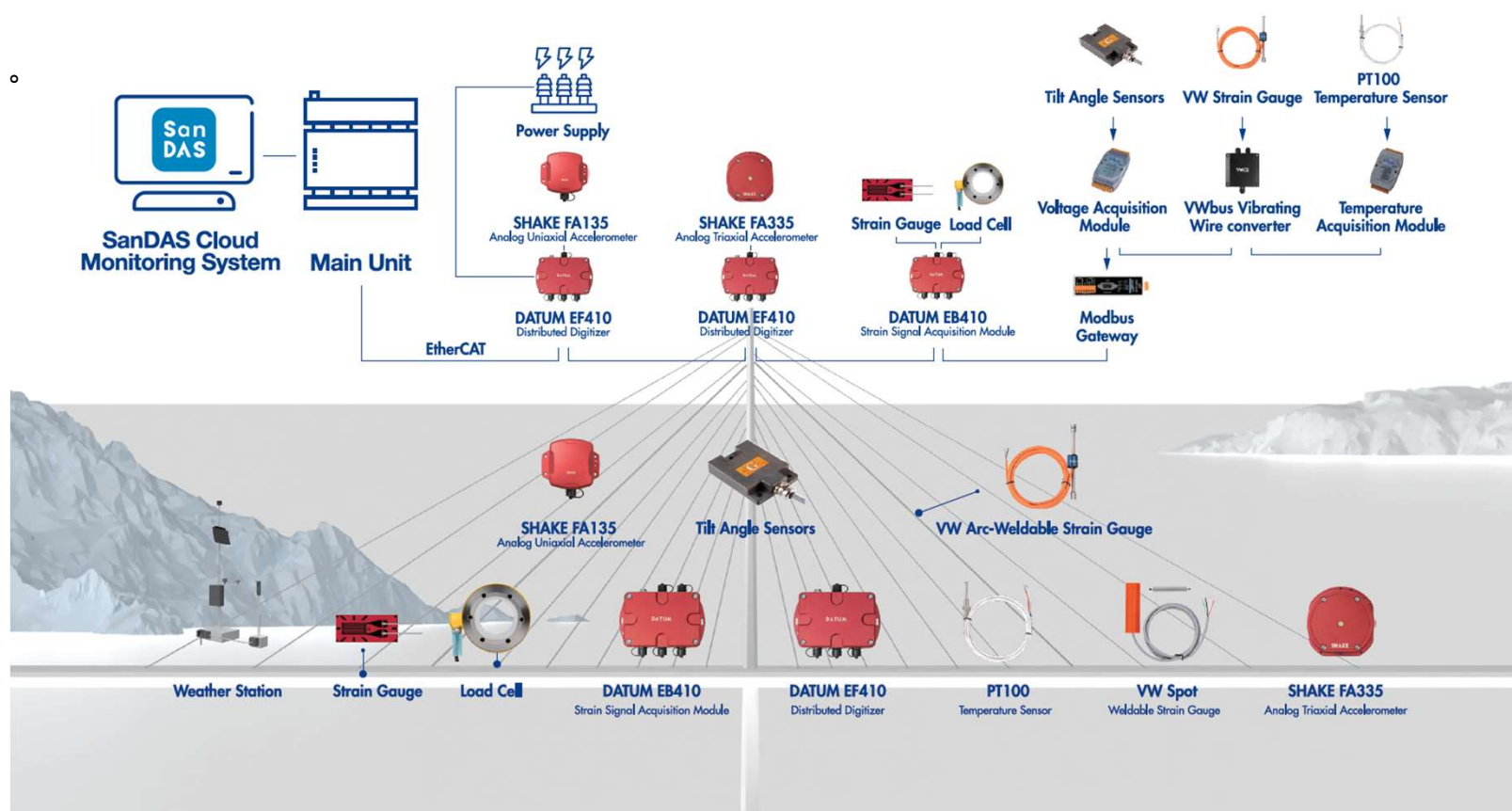
橋梁結構健康監測系統架構
