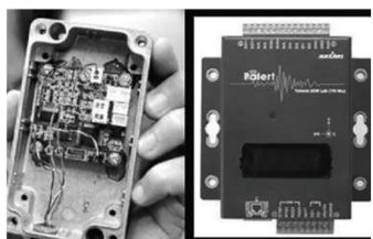
2007 台灣第一套 地震預警系統
